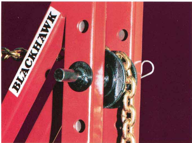
100mm間隔のプリング高さ調整
